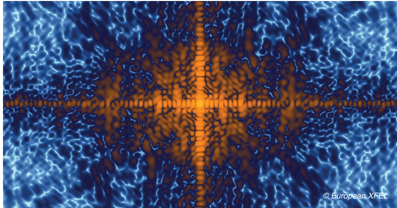
Symulacja obrazu dyfrakcyjnego
