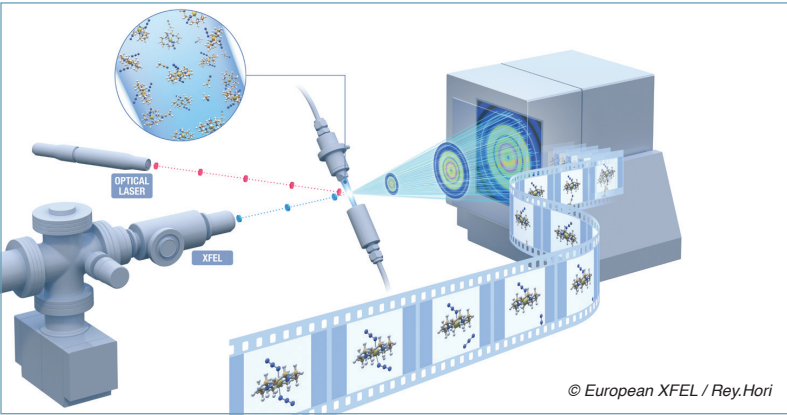
Ultra krótkie błyski promieniowania rentgenowskiego pozwalają robić zdjęcia chwilowych stanów wiązań chemicznych zmieniających się w czasie zachodzenia reakcji. Serie takich zdjęć można następnie wyświetlać jak filmy obrazujące przebieg procesu.
