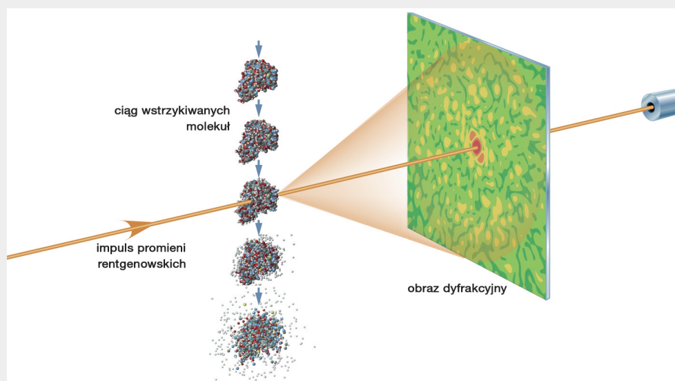
Rys.7 Impuls promieniowania rentgenowskiego z lasera FEL pada na wstrzykniętą biomolekulę. Kamera ustawiona za punktem interakcji rejestruje obraz dyfrakcyjny niosący informację o strukturze molekuli tuż przed jej zniszczeniem. Rejestrując wiele takich obrazów dyfrakcyjnych uzyskanych z kolejnych kopii biomolekuli można będzie zrozumieć budowę molekuli w trzech wymiarach.
