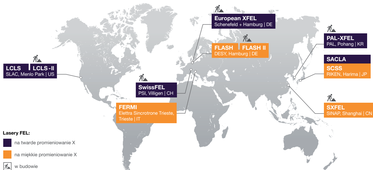
Rys.5 Lasery rentgenowskie na świecie. Obecnie tylko dwa lasery na twarde promieniowanie X (SACLA w Japonii i LCLS w USA) są udostępnione naukowcom.
