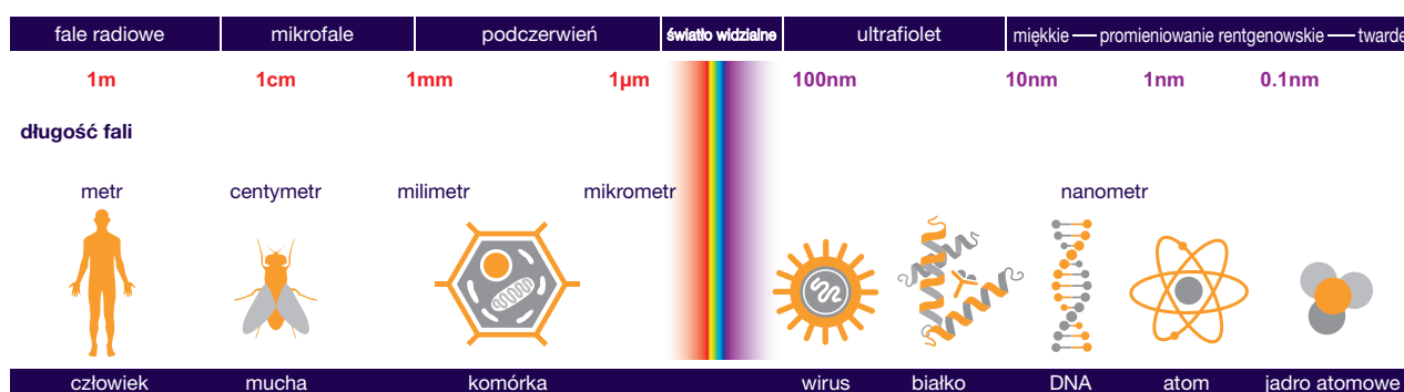
Rys.2 Widmo promieniowania elektromagnetycznego, w którym długości fal w poszczególnych zakresach zilustrowano obiektami o podobnych rozmiarach. Im krótsze fale, tym mniejsze obiekty mogą być obrazowane przez dane promieniowanie.
